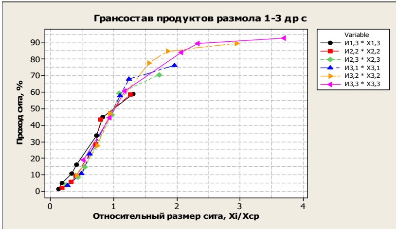
Рисунок 3 – Зависимость величины прохода от относительного размера отверстий сита I, II и III драных системах
