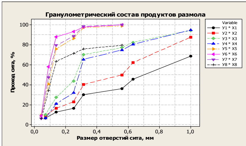
Рисунок 1 – Гранулометрический состав продуктов размола зерна тритикале сорта «Консул», индексами У1-У4 – обозначены драные системы, У5-У8 – размольные системы
