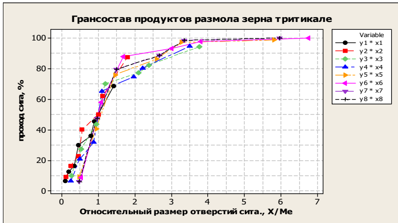
Рисунок 2 – Зависимость величины прохода от относительного размера отверстий сита
